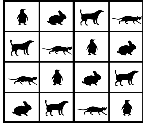
Sudoku 2
