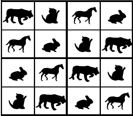
Sudoku 1
