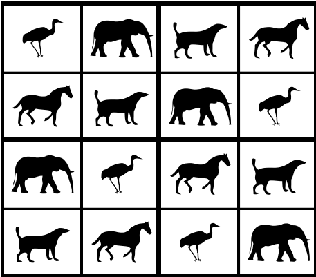
Sudoku 3
