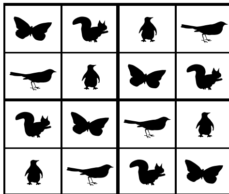
Sudoku 5
