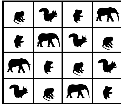
Sudoku 4
